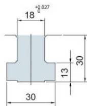
T-Slot
